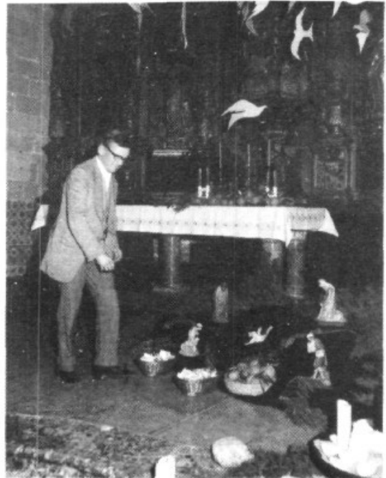
massa vegades)
