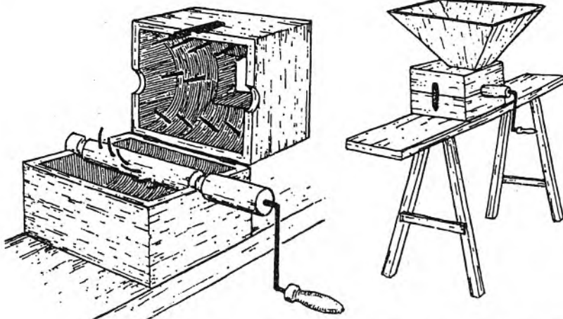
Màquina de capolar figues. Dibuix de Biel Bonnín
