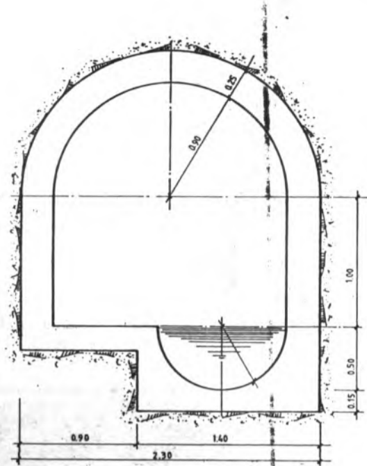
DETALLE SECCION ESTADO ACTUAL COLECTOR GENERAL EN GRAN VIA COLON
