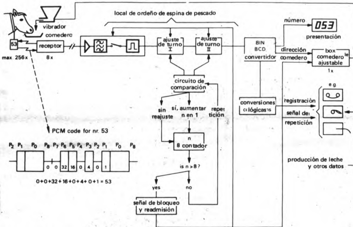
Fig. 2 Diagrama esquemático del sistema de identificación de vacas
