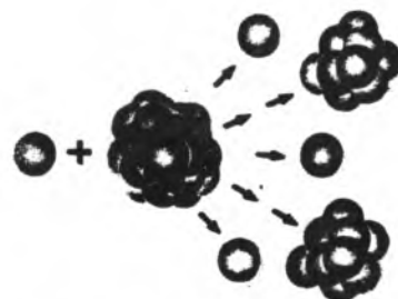
Esquema de una fisión nuclear.
