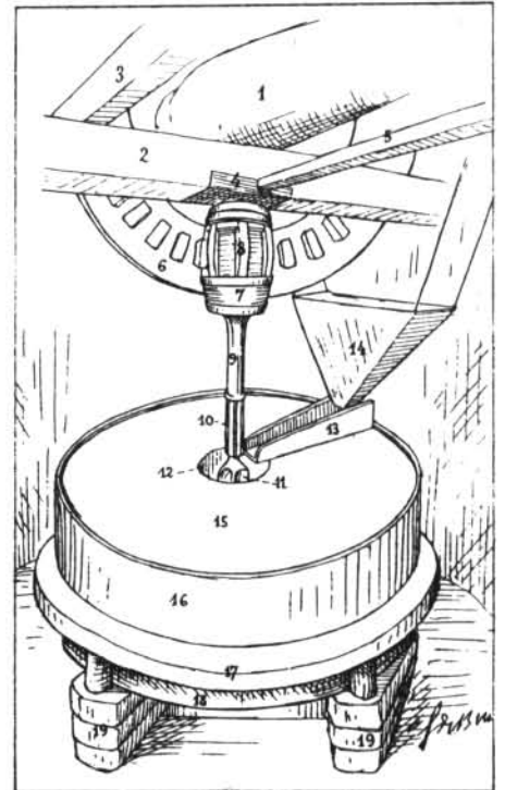
Part superior del mecanisme de les moles d'un molí de vent: 1- arbre; 2- jou; 3- guiera; 4- truvera; 5- estrebador o apitrador; 6- roda; 7- llanterna; 8- braçol; 9- forcada; 10- tecatec; 11- queixals; 12- ull de sa mola; 13- canalet; 14- tremuja o pastereta; 15- mola de damunt; 16- riscla; 17- congrenyets; 18- mola de davall; 19- jasseró.
