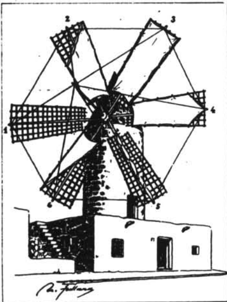
Molí de vent mostrant les diferents maneres de disposar les aspes: 1- desenvelada; 2- escoada; 3- vela plena; 4- escaçada; 5- aplegada; 6- esquarterada.
