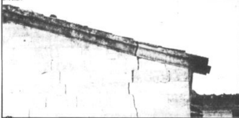
Grietas. Las anchas grietas aparecidas a ambos lados de la capilla del "Roser", y tanto en su parte inferior como superior, amenazan ya la estructura del edificio y reclaman urgentes medidas de reparación.
