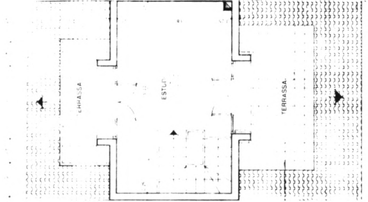
PLANTA PIS 2ª SUP. CONSTRUÏDA PER PLANTA 84.87 M 2 SUP. CONSTRUÏDA PER VIVENDA 28.29 M 2
