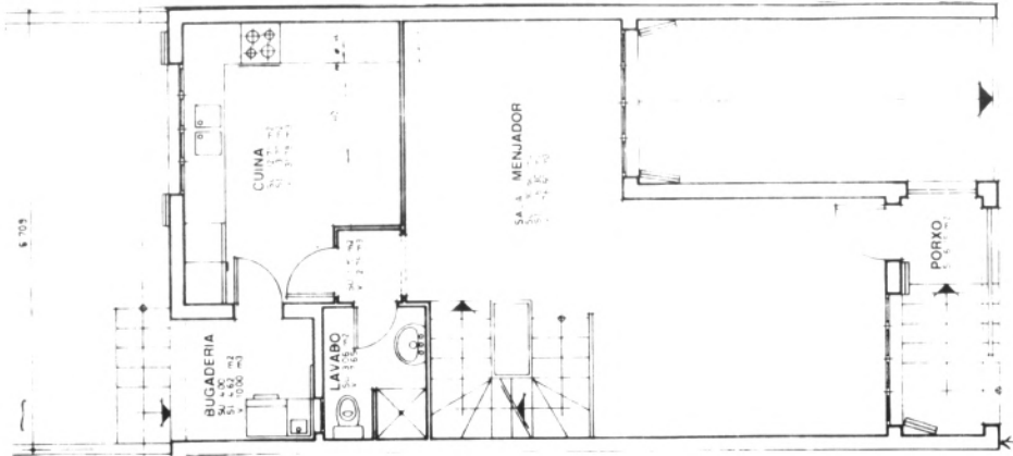
PLANTA BAIXA SUP. CONSTRUÏDA 63.53 M 2
