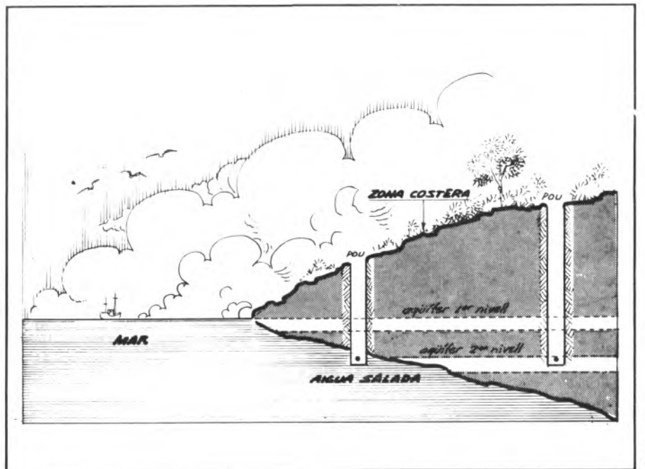
nº 2: Els peus excavats ala zona costera arriben a un primer nivell d'aqüífers, els que s'esgoten abans. Només els pous de l'interior poden arribar a nivells més baixos sense trobar aigua salada
