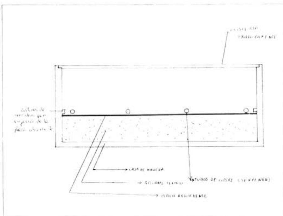
Corte transversal de la placa solar térmica.
