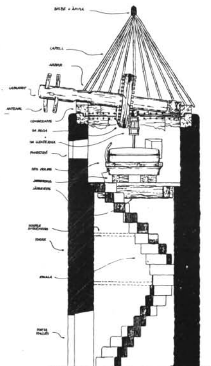
Secció d'un molí; hi ha torres lleugerament còniques
