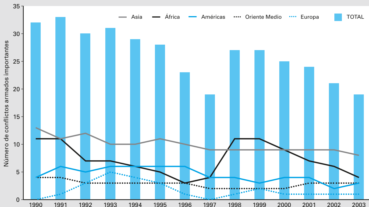
Gráfico 3.2 Dónde se producen los principales conflictos armados
