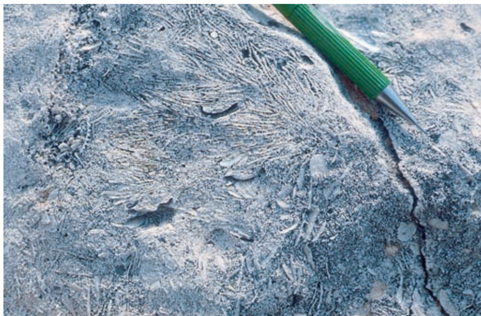
Fig. 4.13. Nivell rudstones d' Heterostegina a cala en Blanes. Representa el sistema transgressiu (TST: Transgressive Systems Tract ) de la Unitat d'Esculls del Tortonian superior-Messinià.
