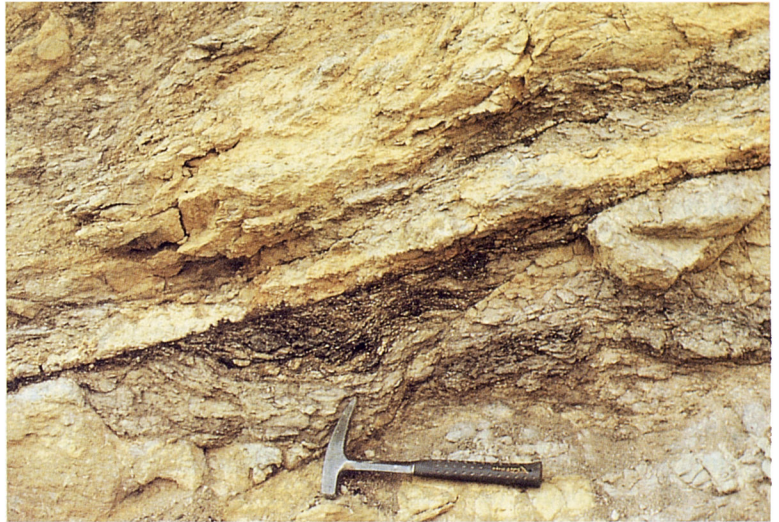
Fig. 8. Prop del Caló des Macs (península septentrional). Encavalcament en els materials margosos de l'Eocè que pinça nivells amb carbó.
