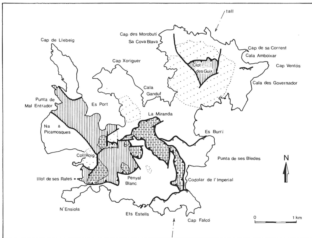
Fig. 5. Esquema estructural de l'illa de Cabrera. Unitat inferior: en blanc els materials mesozoics i puntejat, els eocens. Unitat estructural superior: ratllat, dolomies i bretxes dolomítiques; enrajolat, calcàries oolítiques i algals (SABAT i SANTANACH, 1985).
