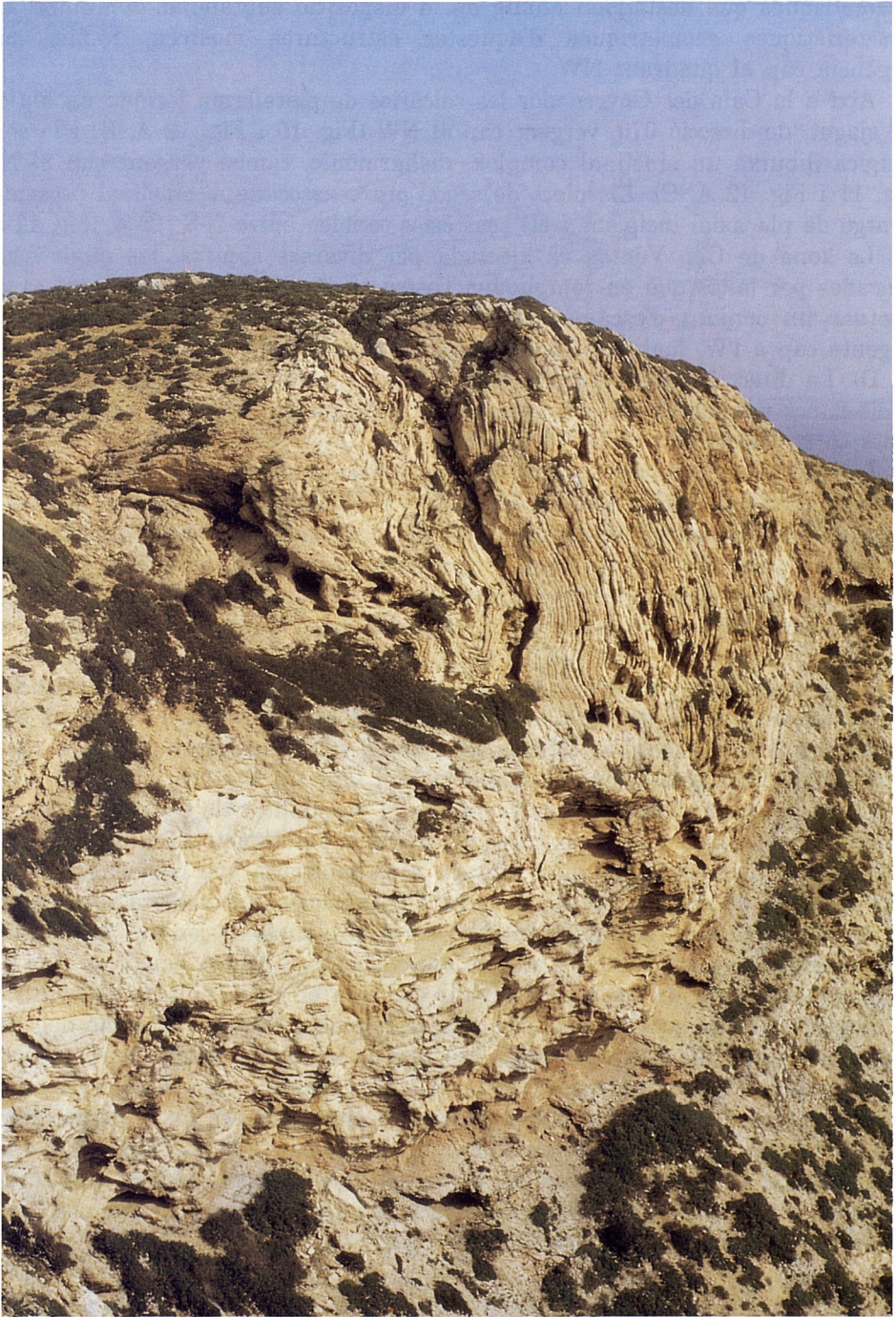
Fig. 11. Sinclinal lleugerament disharmònic i vergent cap al NW que afecta la sèrie pelàgica mesozoica de l'Escala des Governador (península septentrional). Vista presa des del SW.
