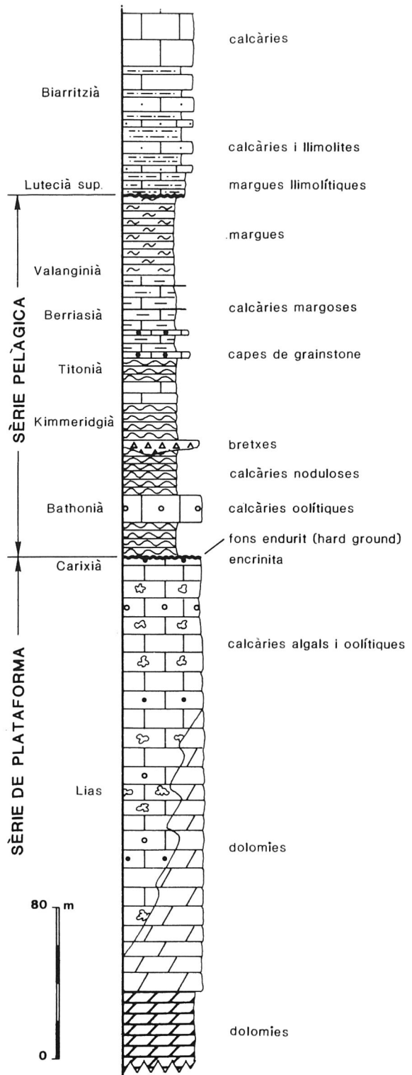
Fig. 1. Columna estratigràfica sintètica de l'illa de Cabrera (SÀBAT i SANTANACH, 1985).
