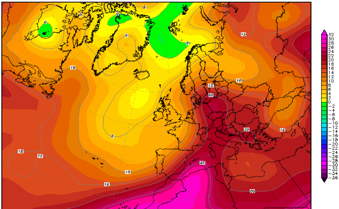
Mapa 62. Anàlisi en superfície del dia 17/07/2007 (00h UTC).
