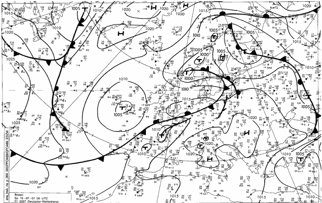
Mapa 57. Anàlisi en superfície del dia 15/07/2007 (00h UTC).
