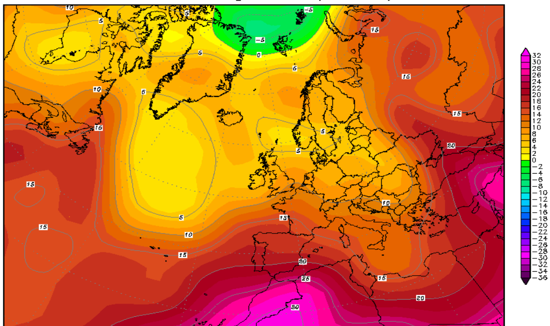
Mapa 52. Anàlisi en superfície del dia 13/07/2007 (00h UTC).
