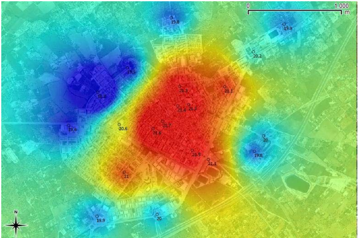
Mapa 35. Isotermes del 11/05/2007 a les 22h 42 min.
