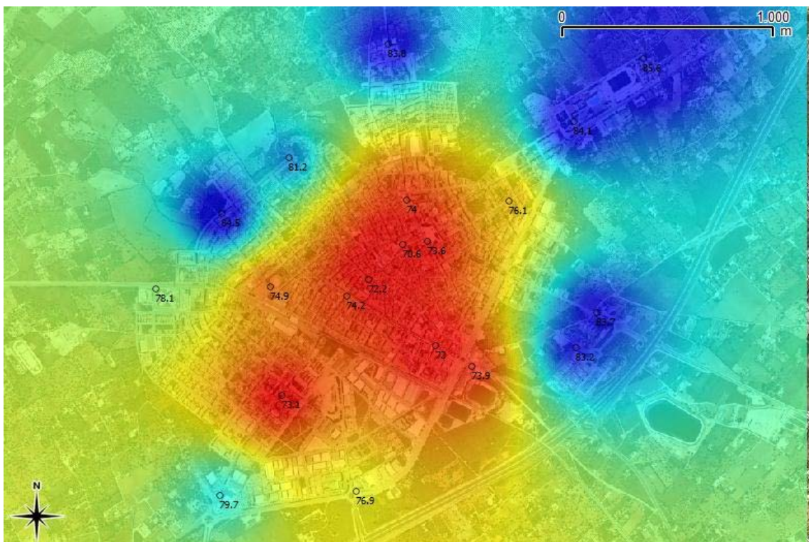
Mapa 115. Isotermes del 13/12/2007 a les 21h 52 min.
