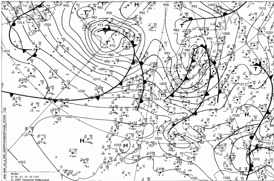
Mapa 7. Anàlisi en superfície del dia 05/01/2007 (00h UTC).
