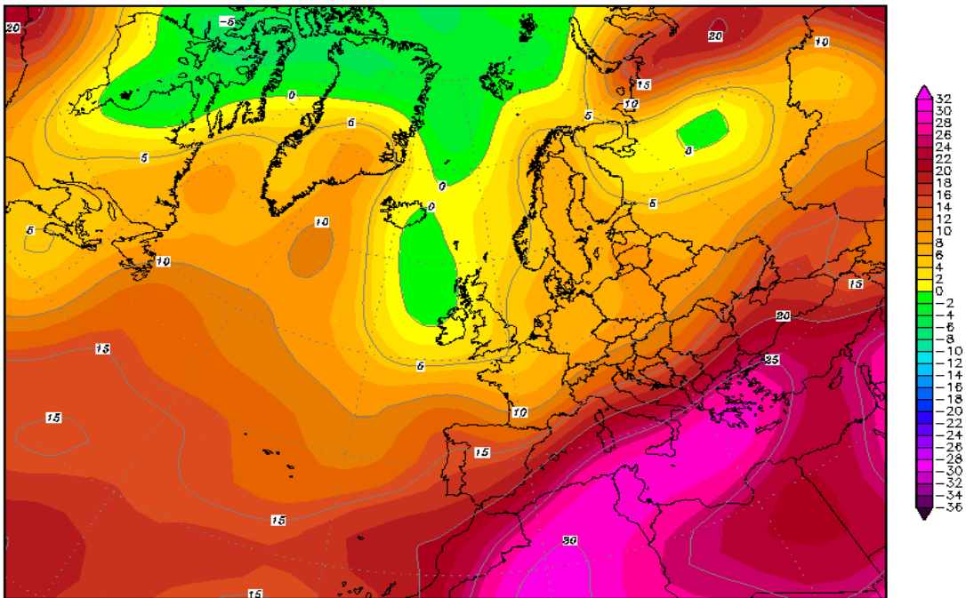
Mapa 42. Anàlisi en superfície del dia 24/06/2007 (00h UTC).
