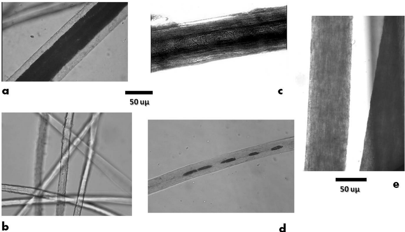
Figura 6. Detalle de los canales medulares por tipos de fibras animales: a) pelo de vicuña; b) lanilla de vicuña (INTA Abra Pampa, Jujuy, Argentina); c) pelo de guanaco; d) lanilla de guanaco (Nevados del Aconquija, Catamarca, Argentina) y e) cabello humano, individuo femenino adulto (sitio PP4, Antofagasta de la Sierra, Argentina). Imágenes tomadas en microscopio óptico a 400 X.
