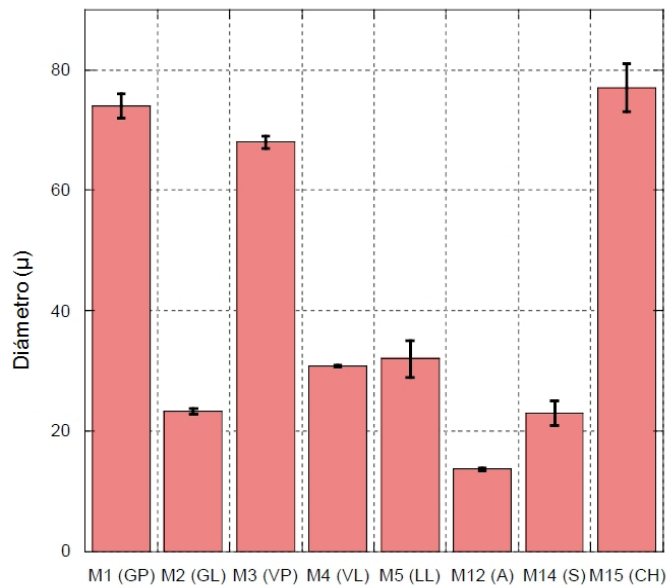
Figura 2. Gráfico comparativo que muestra los valores de media y error estándar de los diámetros ( \mu ) de las fibras/filamentos ensayados.
