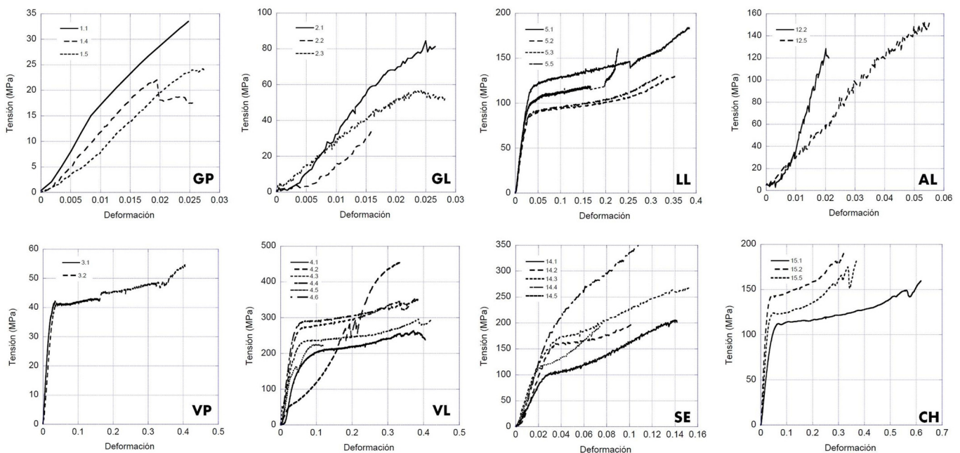
Figura 3. Resultados de los ensayos de tracción fibra/filamento individual: (GP) pelo de guanaco; (GL) lanilla de guanaco; (VP) pelo de vicuña; (VL) lanilla de vicuña; (LL) fibra intermedia de llama; (AL) fibra de algodón; (SE) filamento de seda de lepidóptero y (CH) cabello humano.
