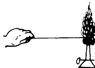
FIGURA 10. Emisión de radiación electromagnética por una sustancia excitada. 9
