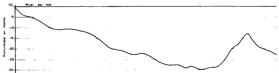
Gràfic 2. Perfil longitudinal de la línia de major fons.
