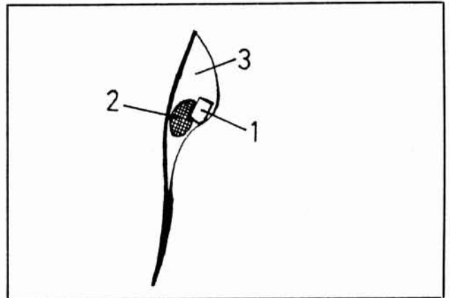
Fig. 6.—Inclusión trifásica, burbuja de gas (3), líquido (2) y cristal de ClNa (1) en una esmeralda de Colombia.
