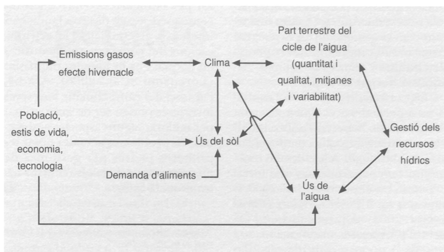
GRÀFICA 2 CONSEQUÈNCIES DE LES ACTIVITATS ANTRÒPIQUES SOBRE ELS RECURSOS D'AIGUA DOLÇA I LLUR GESTIÓ, AMB EL CANVI CLIMÀTIC COM UNA DE LES MÚLTIPLES PRESSIONS (GEICC, 2007B)
