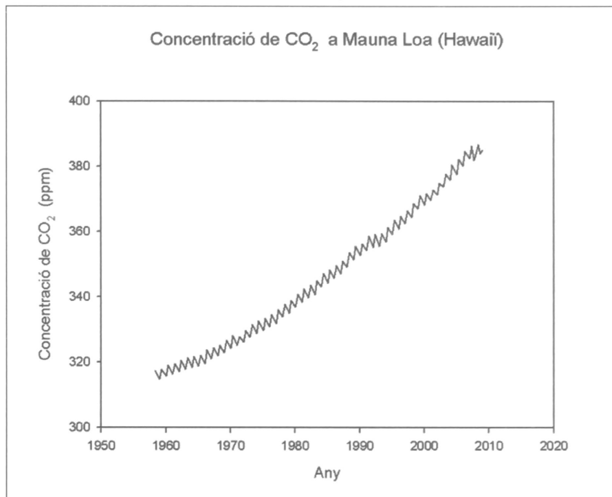
Concentració de diòxid de carboni a l'observatori de Mauna Loa de Hawaii. És el registre més llarg de mesures instrumentals. S'observa el creixement continu, modulats per la variació estacional, de la concentració de \text{CO}_2 a l'atmosfera. Font (Elaboració pròpia a partir de dades de la NOAA: www.esrl.noaa.gov/gmd/ccgg/trends/ )
