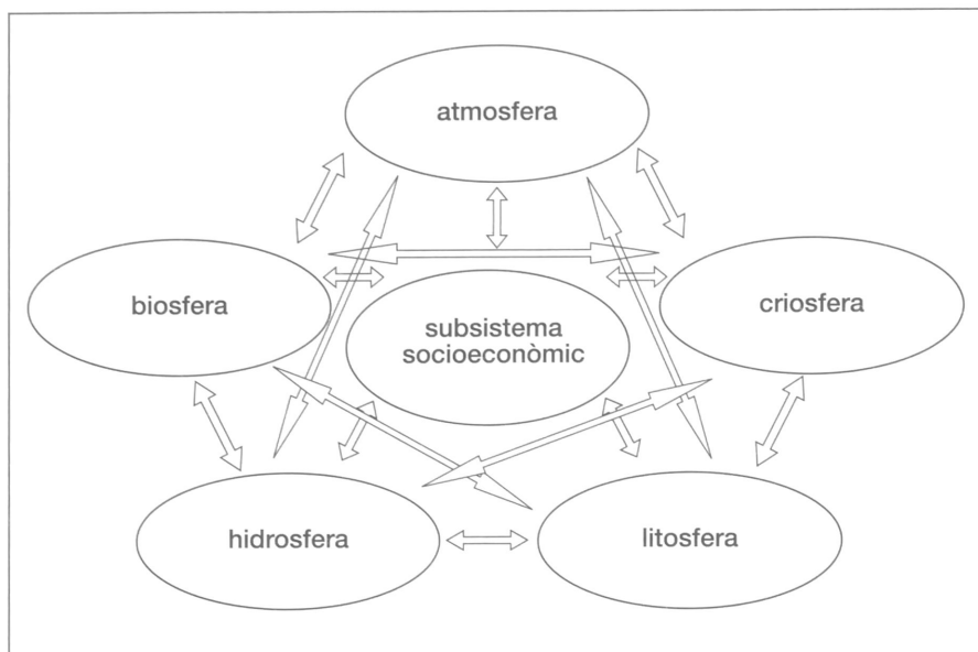
GRÀFICA 1 COMPONENTS DEL SISTEMA CLIMÀTIC
