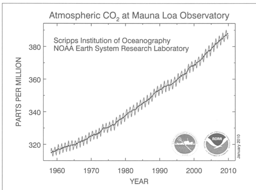
GRÀFICA 2 EVOLUCIÓ DE LA CONCENTRACIÓ DE CO 2 A L'OBSERVATORI DE MAUNA LOA (HAWAII) DES DEL 1958 FINS AL 2009
