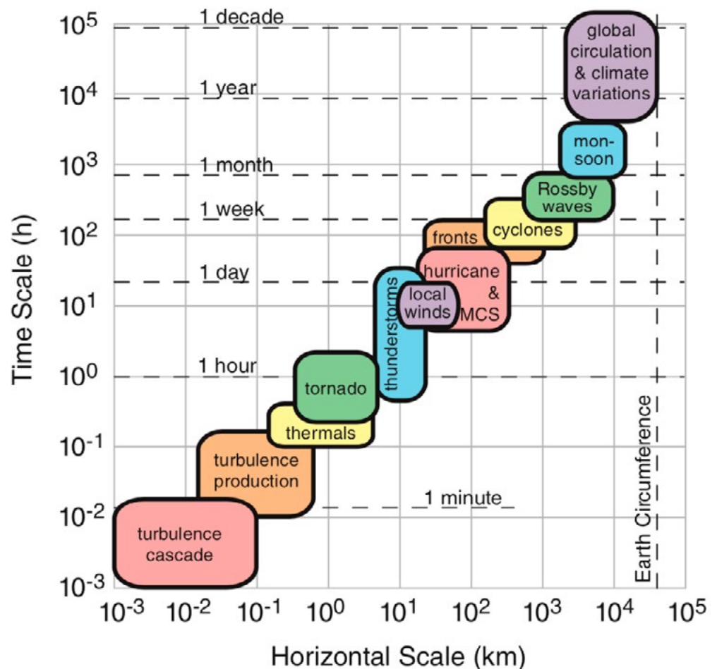
Diagrama d'escalas horitzontals i temporals de les circulacions atmosfèriques (font: Stull 2017)
