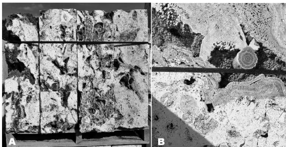
Figura 8. Marès tipus T 2 de la pedrera de sa Màniga: A. Marès brescat comercialitzat amb el nom de «pedra fòssil»; B. Detall on es pot observar la carstificació de les colònies de corall Porites i el posterior rebliment per microespeleotemes.
