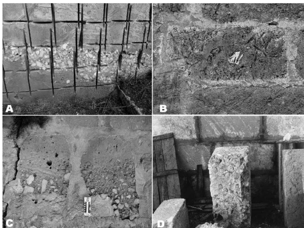
Figura 4. A. Nivell de còdols arrodonits polimíctics (platja) a la base de les pedreres de Son Mulet; B. Gasteròpode Persististrombus coronatus inclòs dins una peça de marès de la zona de Son Mulet – Son Fullana (parament exterior de la casa del cap de cantó del carrer d'Antoni Maura amb el carrer d'Antoni Garcias, a Lluçmajor); C i D. Còdols angulosos monomíctics priabonians (eocè) inclosos dins peces de marès tallades de la base de la pedrera de Galdent.
