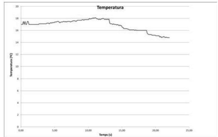
Fig. 19 Gràfica de la variació de temperatura
