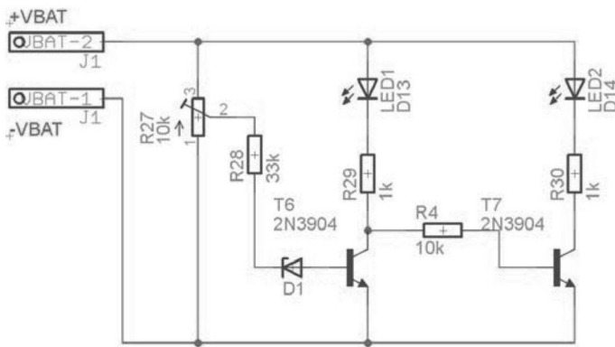
Fig. 6 Disseny esquemàtic de l'indicador de bateries
