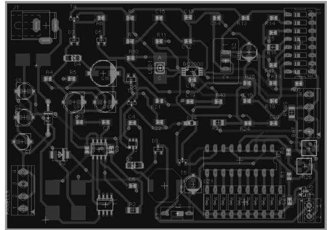
Fig. 7 Layout del mòdul d'alimentació
