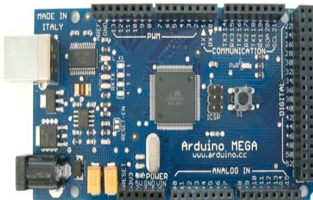
Figura 3, Arduino Mega
