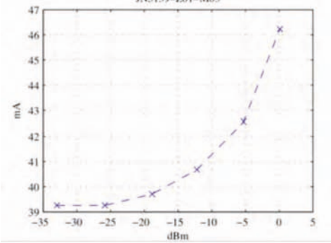
Fig. 9 Comparativa de la P_{Tx} versus el consum de corrent dels mòduls JN5139-Z01-M03 de Jennic.
