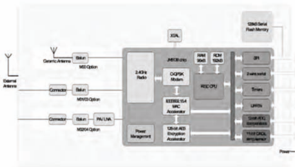
Fig. 3 Esquema dels elements que formen un mòdul JN5139-Z01-M03.
