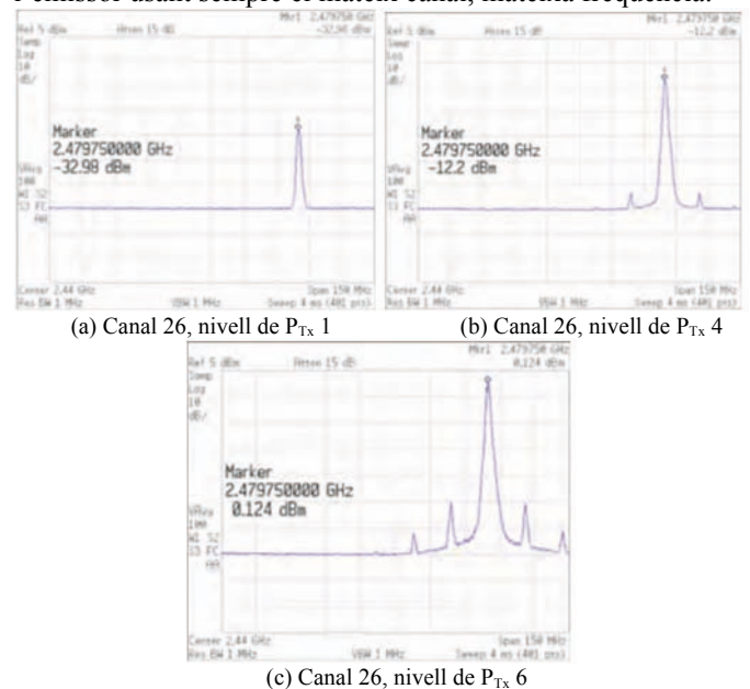
Fig. 5 Captures de l'espectre de sortida del senyal generat pel mòdul JN5139-Z01-M03 a diferents nivells de P_{Tx}
