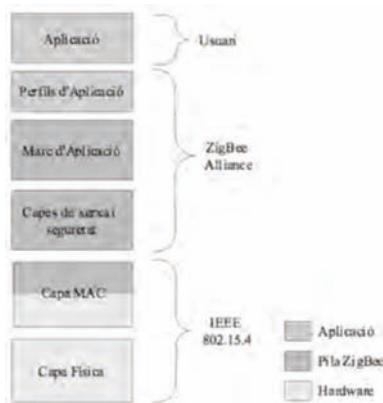
Fig. 1 Pila de protocols on es poden veure els nivell definits per cada un dels diferents estàndards IEEE802.15.4 i ZigBee.
