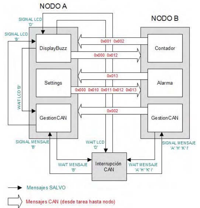
Fig. 4 Esquema básico
