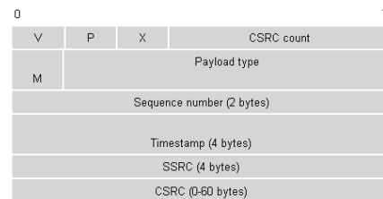
Figura 1. Capçalera del paquet RTP.
