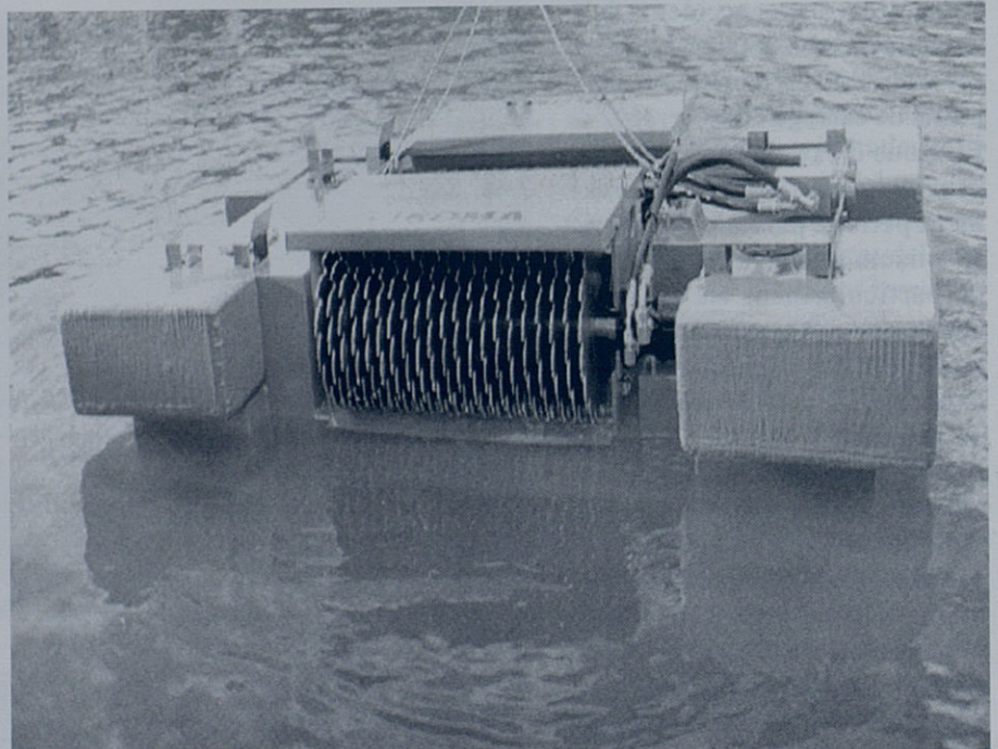
Les accions externes adreçades a minimitzar els efectes dels hidrocarburs es denomina pla de contingència.
