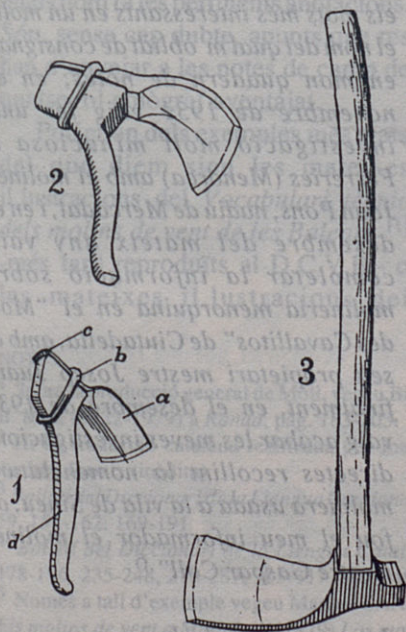
1, alxa dreta;—2, alxa girada;—3, alxa de peu. a, pala;—b, esclop;—c, coa;—d, màneg (en la terminologia d'Eivissa).
