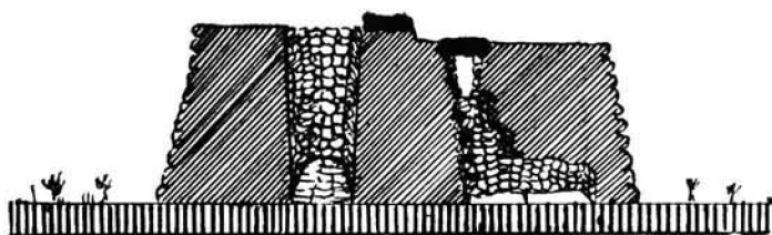
Fig. 2. Sección por D E 1 : 200
