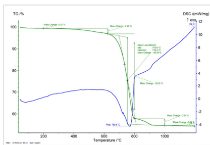
Fig. 20. STA-diagram of the sample S2. Fig. 20. Diagrama STA de la mostra S2.
