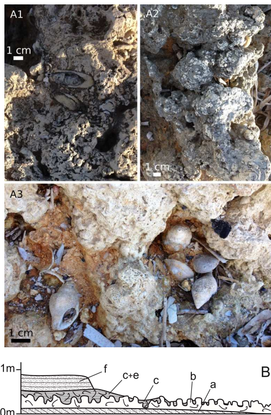
Fig. 11. Torrent de son Real. A: Detalls dels tapissos algal, A1: Tapís algal perforat per litòfags; A2: Detall del tapís menys erosionat, on s'observen les morfologies globoses de les algues incrustants; A3: Rebliment dels espais entre els doms algal amb sorres i llims vermellosos, i espècies termòfiles com Gemophos viverratus (Kiener, 1834). B: Tall estratigràfic S-N, modificat de Vicens (2015), a: Eolianita del Riss; b: Bioconstruccions domals d'algues coral·linals incrustants amb fauna marina de l'OISS-5e; c: Llims vermellosos (més arenosos com més a prop de la costa) amb fauna marina de l'OISS-5e; e: Llims vermellosos; f: Eolianita. Nota: Aquest tall no inclou la platja de l'OISS-5a que figura Vicens (2015) amb la unitat 'd' a causa de que en la secció aquí referenciada (a uns 150 m al NE de la desembocadura del torrent) aquesta és absent.
