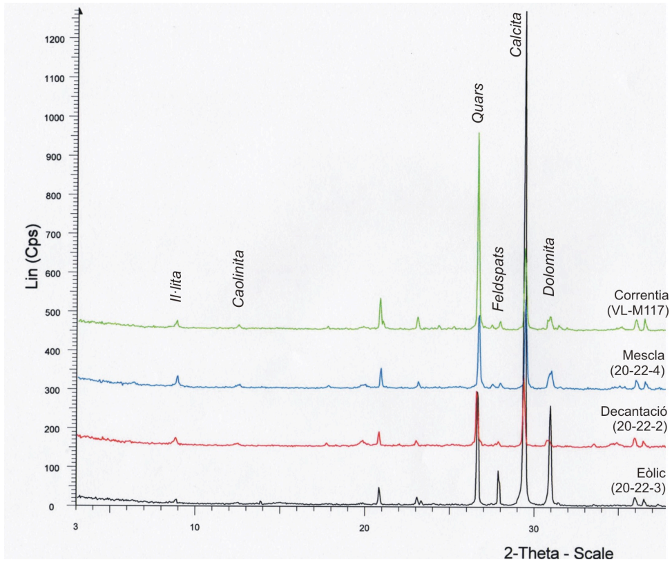
Fig. 3. Diffractogrames de raigs-X de mostres representatives de les fàcies presents a la galeria del Tragus de la cova des Pas de Vallgornera.
