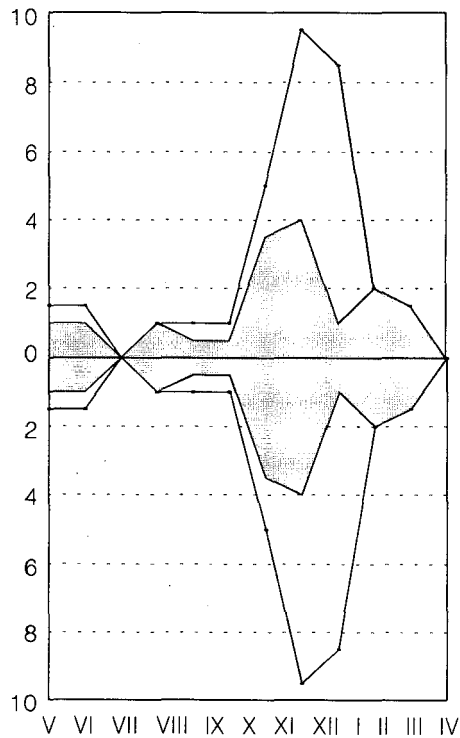
Fig. 5. Adultos (especies -sombreado- y individuos) capturados en Ses Puntos (pinar).
