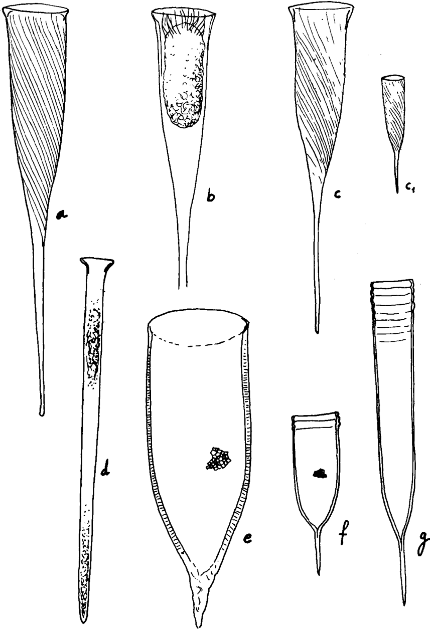
Fig. 10-a,b: Rhabdonella conica Fig. 10-c: Rhabdonella spiralis Fig. 10-d: Salpingella attenuata
