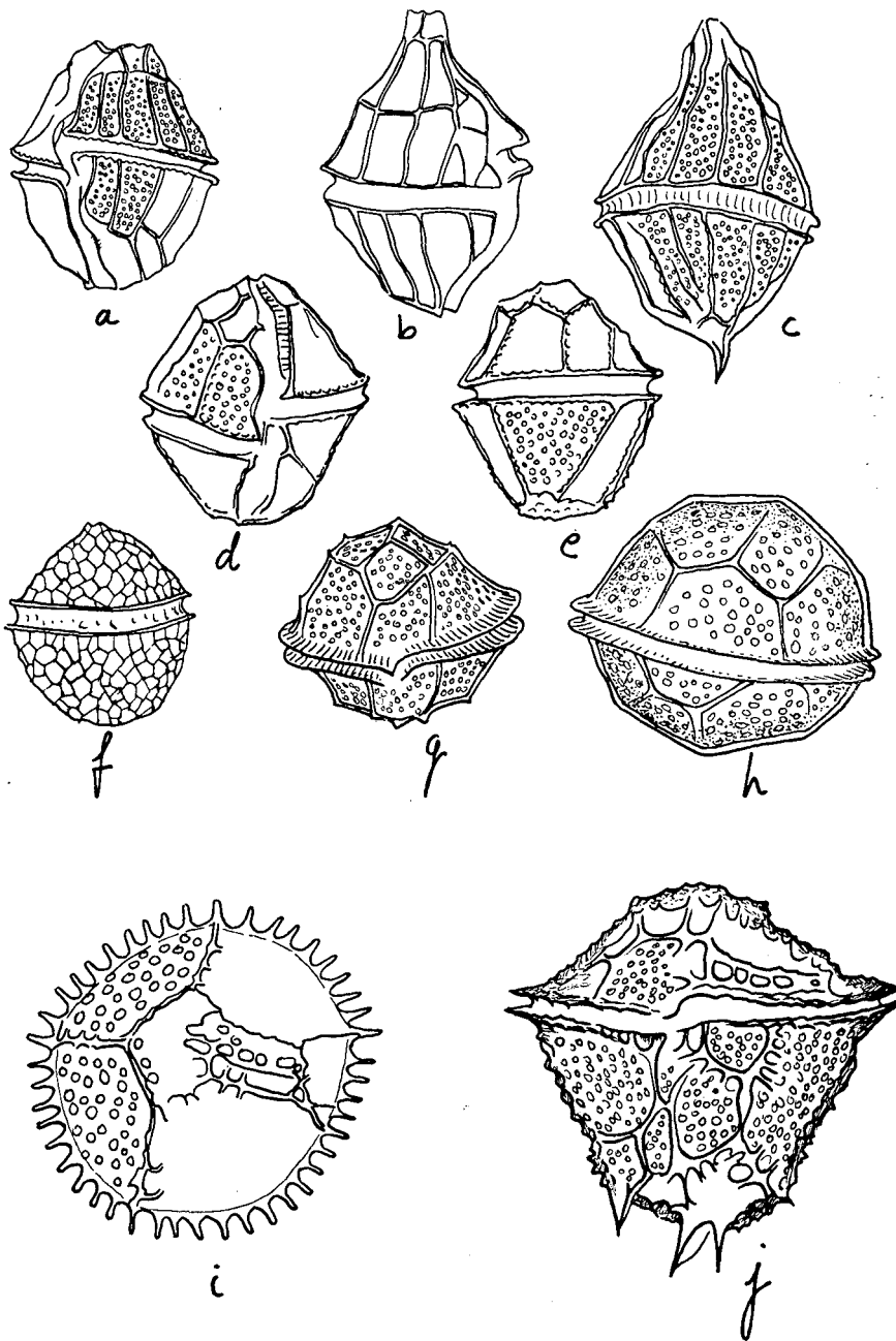
Fig. 8-a,b: Gonyalux spinifera Fig. 8-c: Gonyalux polygramma Fig. 8-d,e: Gonyalux polyedra Fig. 8-f: Protoceratium reticulatum
