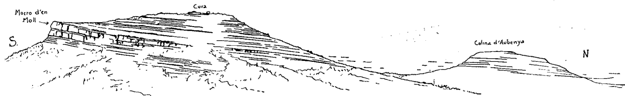
Fig. 4.—La porción Este de la montaña de Randa y la colina de Aubanya, mostrando la suave inclinación de sus estratos hacia el Norte.
