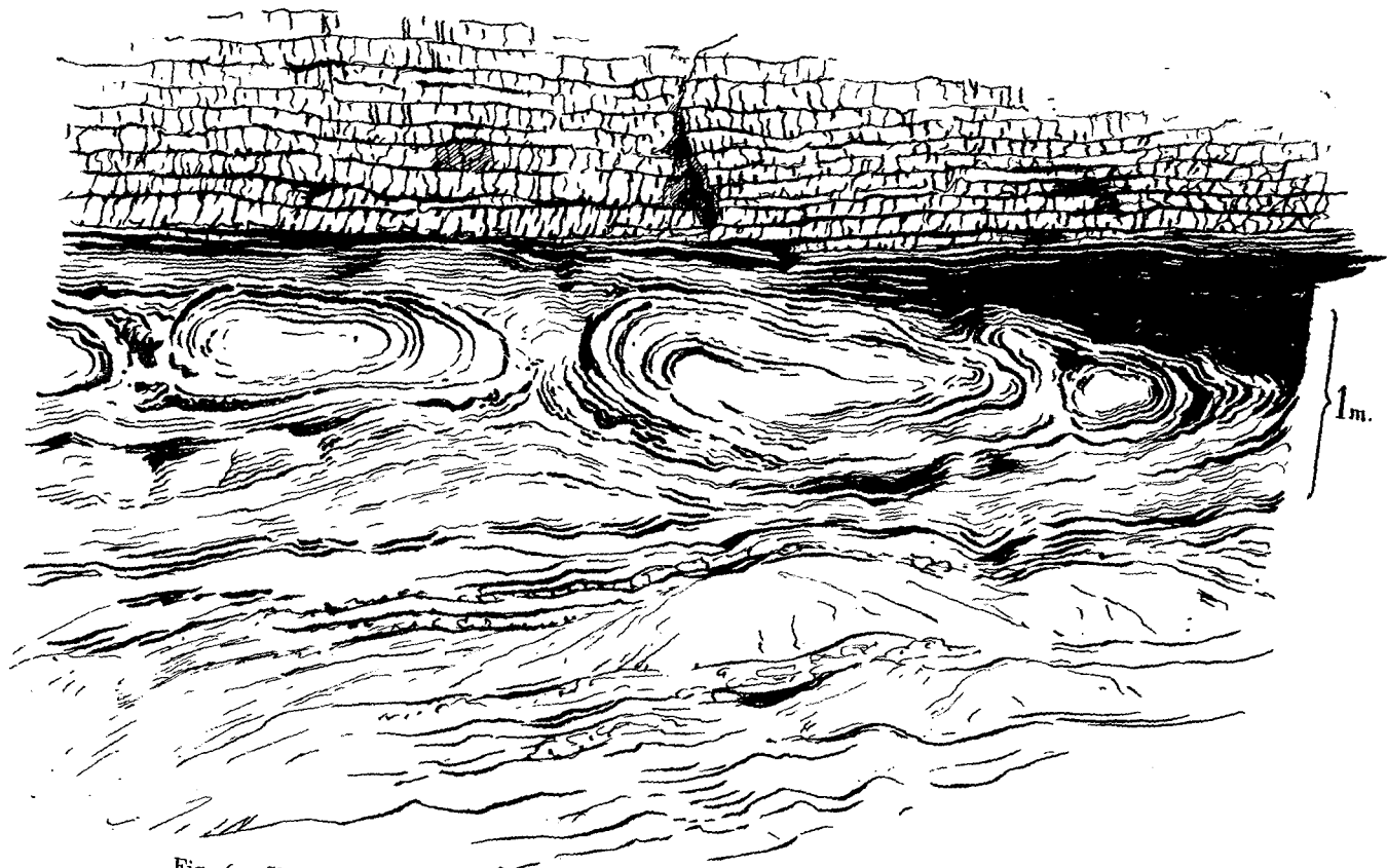
Fig. 6.—Slumping, en las margas burdigalenses, junto a la Ermita de Gracia. Sobre ellas descansan las potentes series calizas, detrítico-zoogenas, con intensas diaclasas. Dirección, N.-NO.
