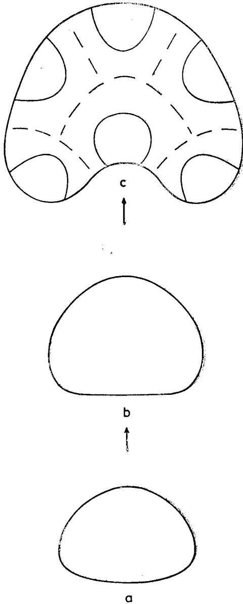
Fig. 23: La différenciation de la section de Psychoceras laeve laeve Math. v. fig. 22, 10/1.
