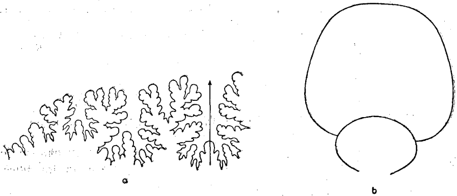
Fig. 9: E. (Eogaudryceras) muntaneri Wiedm. Holotype, MSHNB A 92c, Albien de Son Suremeta. a: ligne suturale, 5/1. b: section du tour, 4/1.
