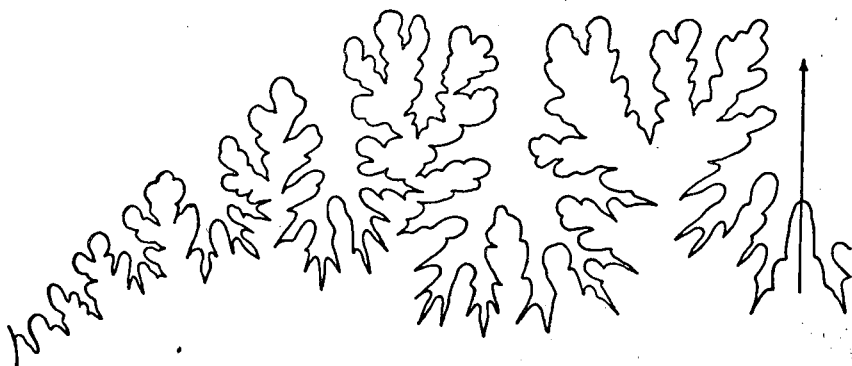
Fig. 11: Ligne suturale de K. (Kossmatella) sublaevis sublaevis Wiedm. Holotype, MHNG Wi «UAM»/1, Albien de La Goudinière. 10/1.
