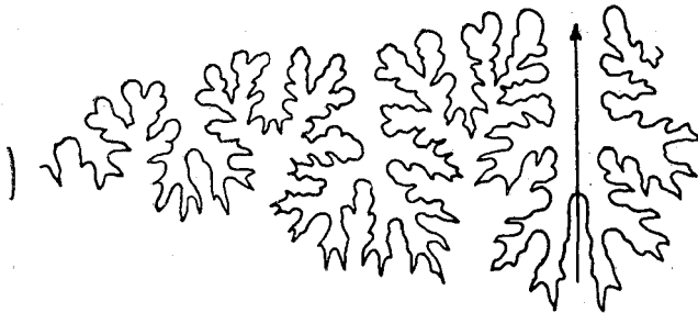
Fig. 14: Kossm. (Cuderianites?) binammata Wiedm. a: Holotype, MSHNB A 69a, section du tour, 4/1; b: Paratype, MSHNB A 69d, ligne suturale, 10/1. Albien de Son Vida.
