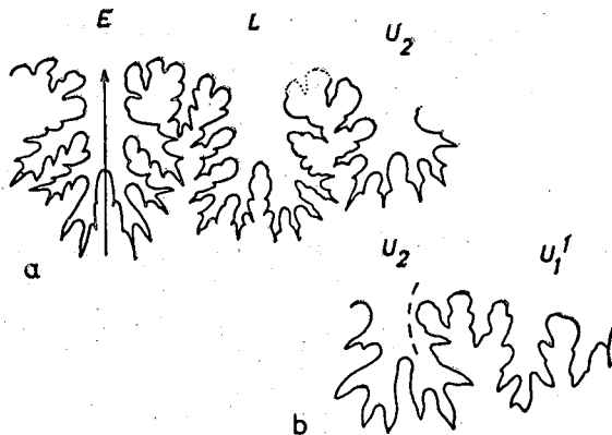
Fig. 16: Jauberticeras? majorcense Wiedm. a: ligne suturale de l'holotype, GPIT Ce 1220/18, 10/1. b: lobes ombilicaux du paratypoïde GPIT Ce 1220/19, 20/1. Marnes de la Cala Blanca.
