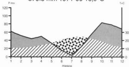
AEROPORT DE MENORCA 570,5 mm 1971-00 16,9°C
