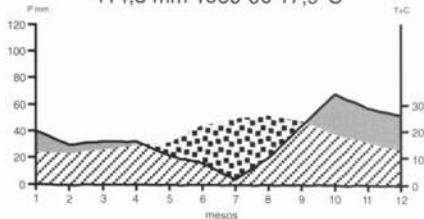
AEROPORT D'IVISSA 414,5 mm 1960-00 17,9°C
