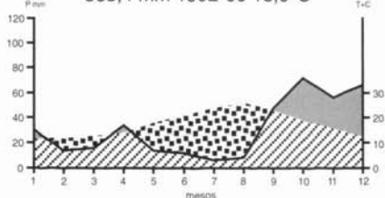
CABRERA 368,4 mm 1992-00 18,0°C
