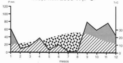
AEROPORT DE MENORCA 419,8 mm 2000 17,7°C
