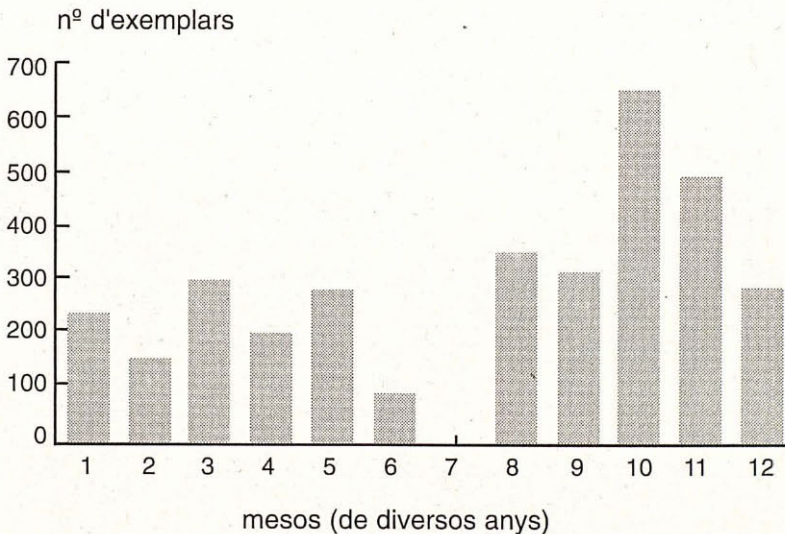
Figura I. Nombre màxim de tiririlo camanegra ( Charadrius alexandrinus ) al Salobrar de Campos (se representen els màxims mensuals, no necessàriament del mateix any, durant el període 1988-1996).
