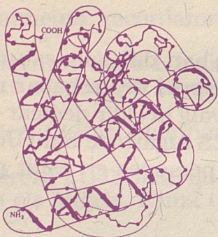
Estructura de la mioglobina por rayos X.
