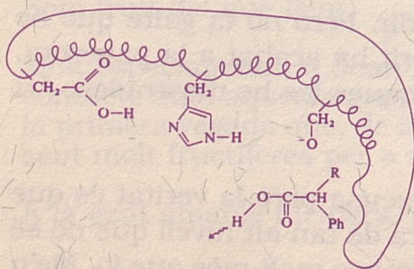
Liberación de ácido carboxílico
