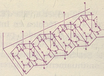
Estructura \beta , o plegada, de las proteínas
