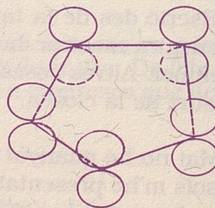
Orbitales atómicos \pi del ciclopentadienillo
