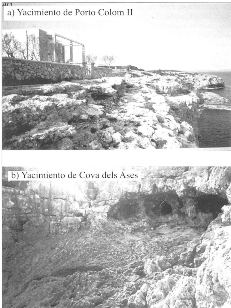
Figura 4. En las costas de erosión encontramos mayoritariamente trampas sedimentarias (a y b) plataformas elevadas (a y b) o afloramientos sobre sistemas dunares fósiles adosados a la base del acantilado (b). Los impactos antrópicos (4a) no les afectan del mismo modo que a los situados en costas bajas.
