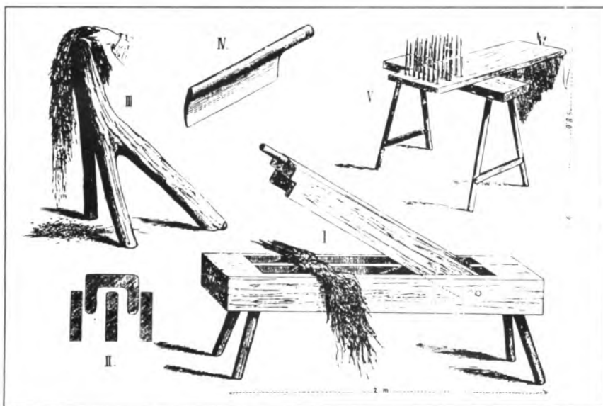
Figura 1. Eines per treballar el cànem. I: Trencador. II: Secció d'un trencador. III: Tribessos. IV: Espadella. V: Puats. Extret de Las Baleares descritas por la palabra y el dibujo , de l'Arxiduc.
