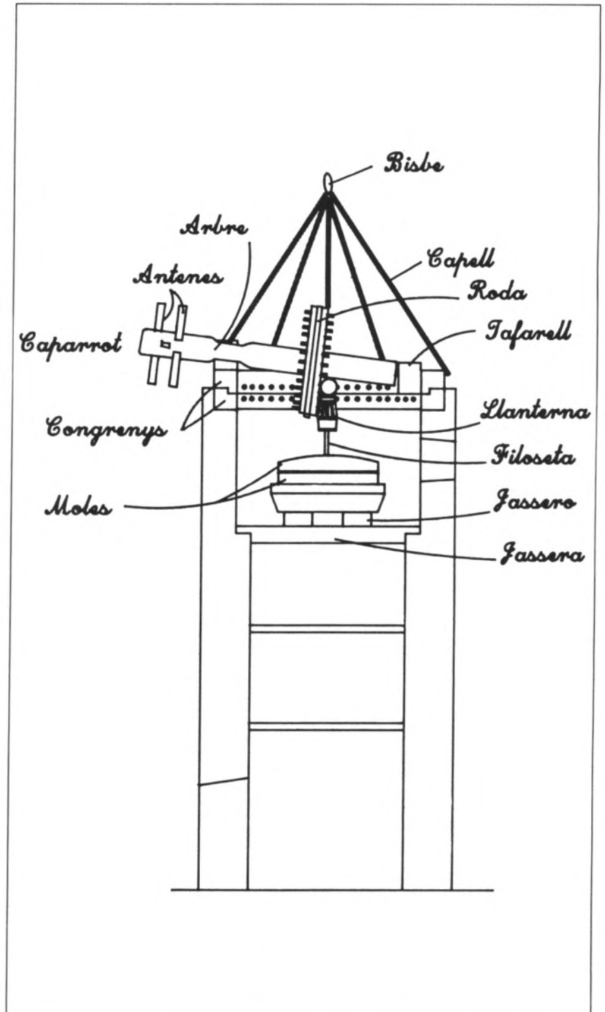
Tall transversal d'un molí de vent fariner, amb tots els seus elements.
