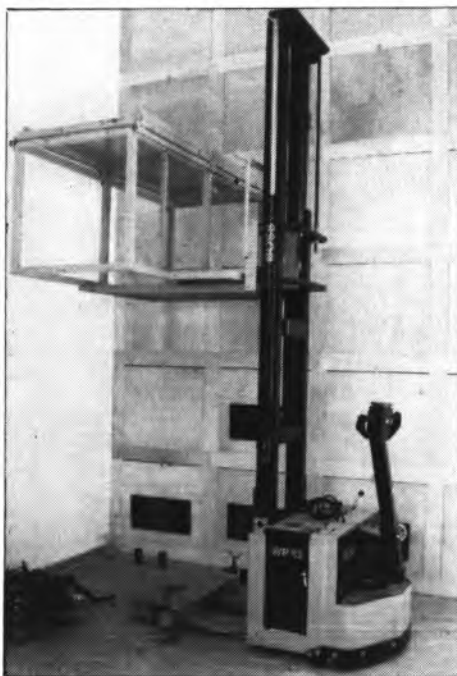
La máquina elevadora para la colocación de féretros
