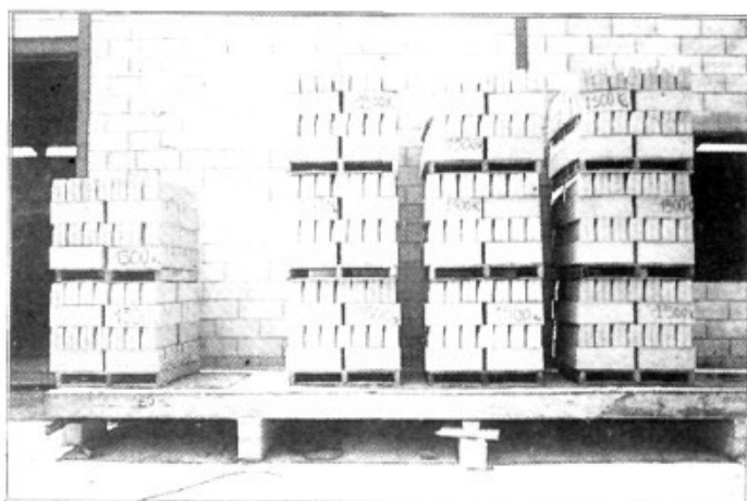
Realización de una prueba de carga
