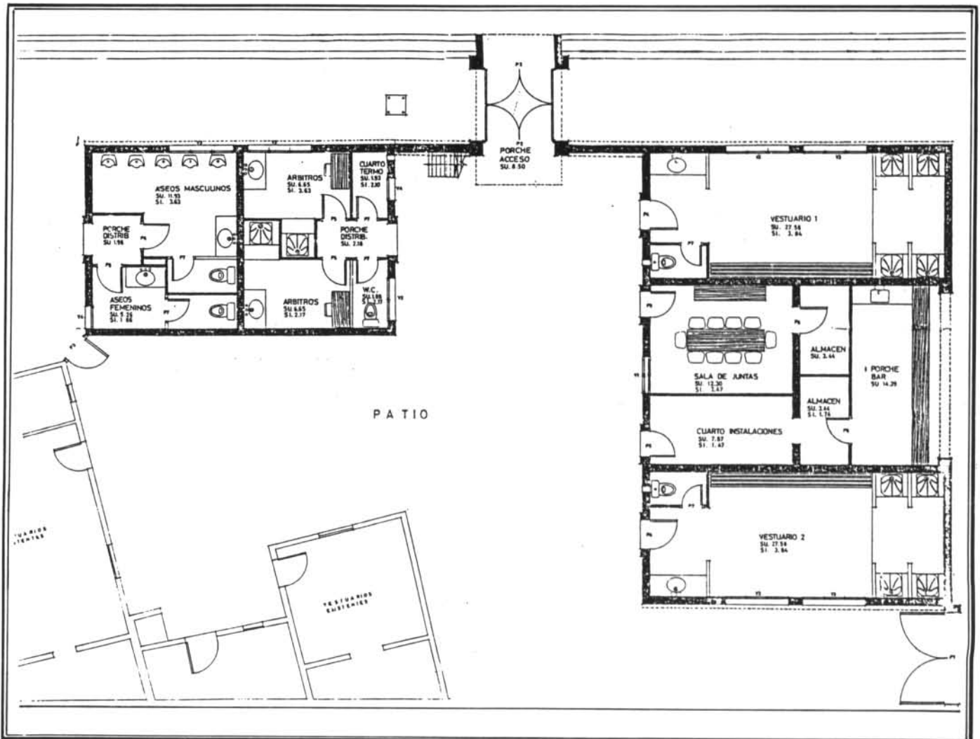
Plànol detallat i complet dels nous vestuaris del camp de futbol "Es Revolt"
