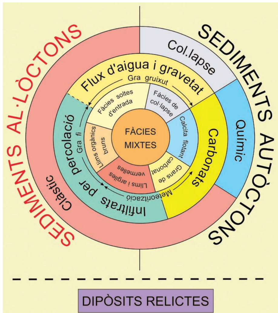
Figura 11: Fàcies sedimentàries i processos implicats en les cavitats litorals de les Illes Balears (modificat de FORNÓS et al. , 2009).
