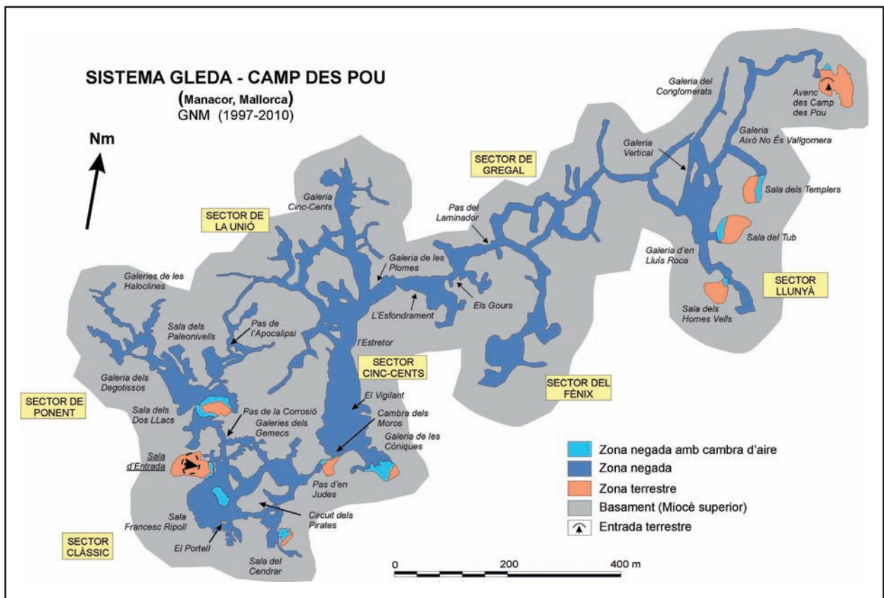
Figura 12: Topografia del sistema Gleda-Camp des Pou (Manacor).
