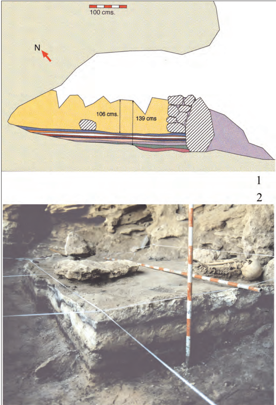
Fig. 3. Sección trasversal de la cueva y de la secuencia estratigráfica (1). Registro sedimentario objeto de estudio (2).
