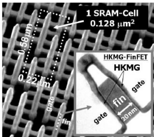
Fig. 8 Parte del diseño de una memoria SRAM con transistores FinFET.
