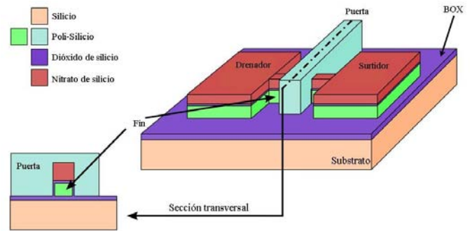
Fig. 2 Estructura básica.
